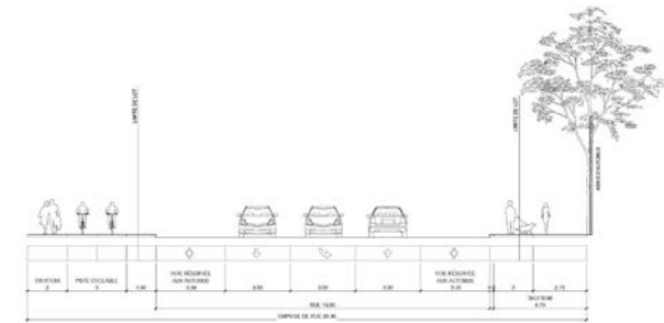
Coupe de rue D-D' proposée pour l'option no1.
